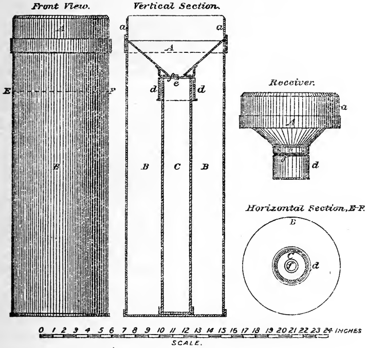
FIG. 1.—Rain gage.
